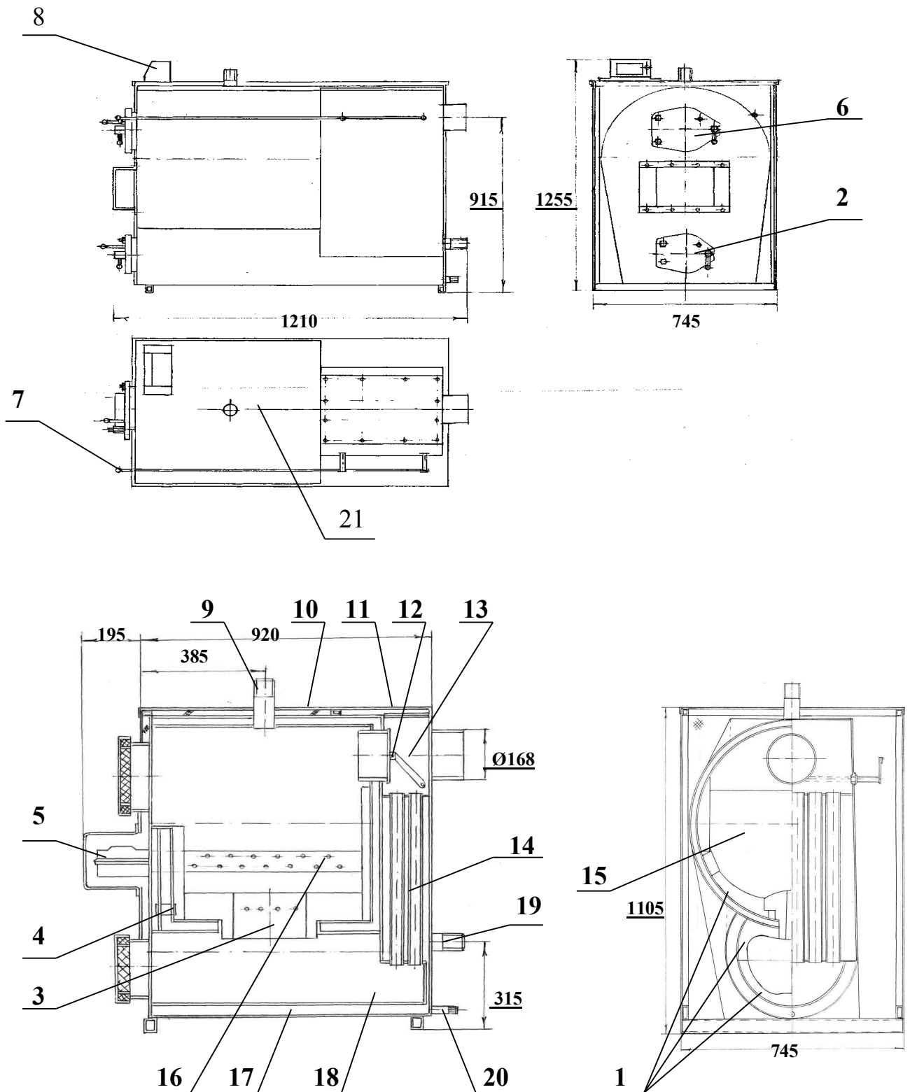
Рисунок 1. Устройство котла. Общий вид, продольный и поперечный разрез.
