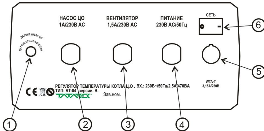
Рисунок 3. Задняя панель регулятора.
